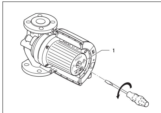
Рис. 6.1 Откачка воздуха из насоса
