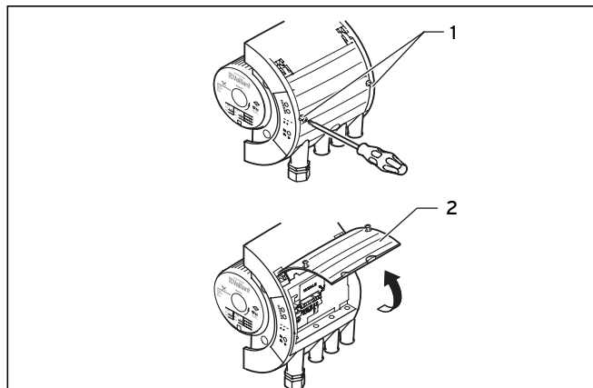
Рис. 4.10 Монтаж модуля GENI
