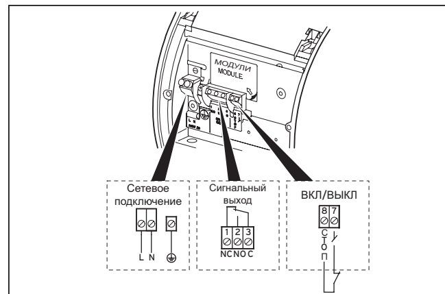
Рис. 5.4 Схема электрических соединений для насосов всех типов
