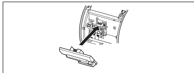
Рис. 4.11 Применение модуля GENI
