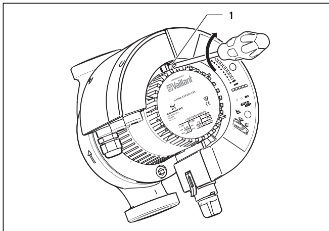
Рис 4.8 Закрепление модуля GENI
