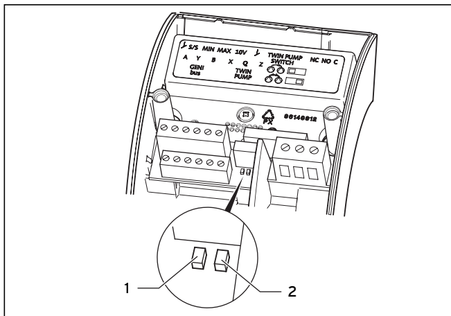
Рис. 9.1 Проверка модуля Geni
