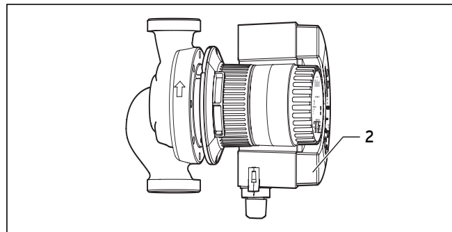
Рис. 4.3 Вытаскивание статора и головки насоса
