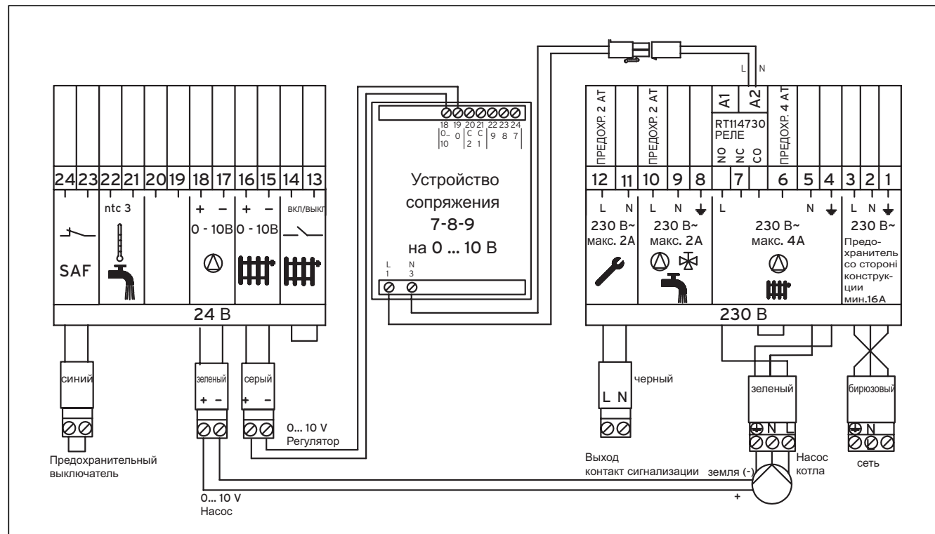
Рис. 5.3 Электрическая схема подключений
