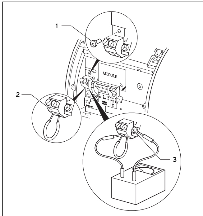
Рис. 10.3 Проверка сопротивления изоляции
