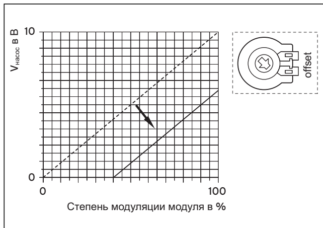
Рис 6.3 Положение до упора влево потенциометра „offset“
