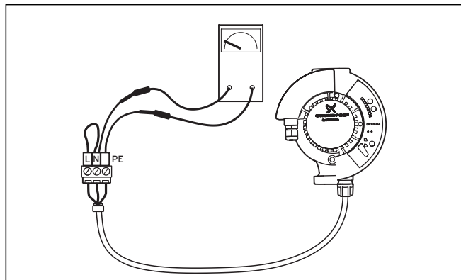
Рис. 10.1 Проверка сопротивления изоляции
