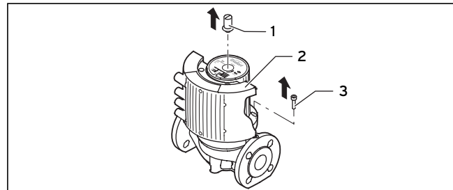
Рис. 4.5 Отвинчивание корпуса статора
