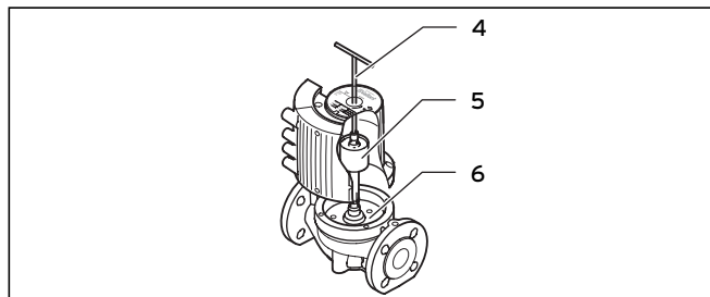
Рис. 4.6 Изменение положение клеммной коробки
