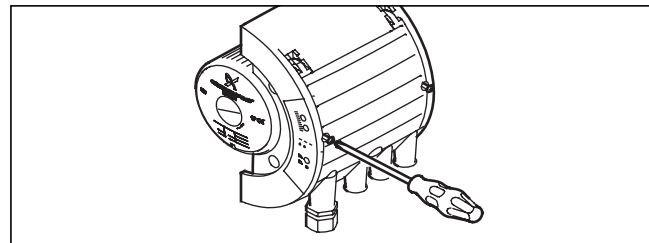
Рис. 5.1 Откручивание крышки клеммной коробки
