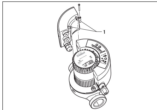
Рис 4.7 Монтаж конструктивного модуля GENI
