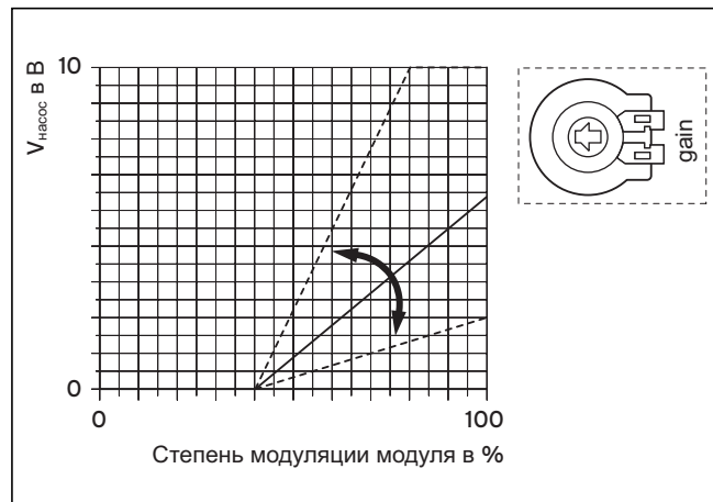
Рис. 6.2 Среднее положение потенциометра „gain“
