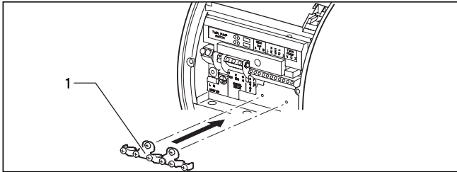
Рис. 4.13 Установка кабельных соединений
