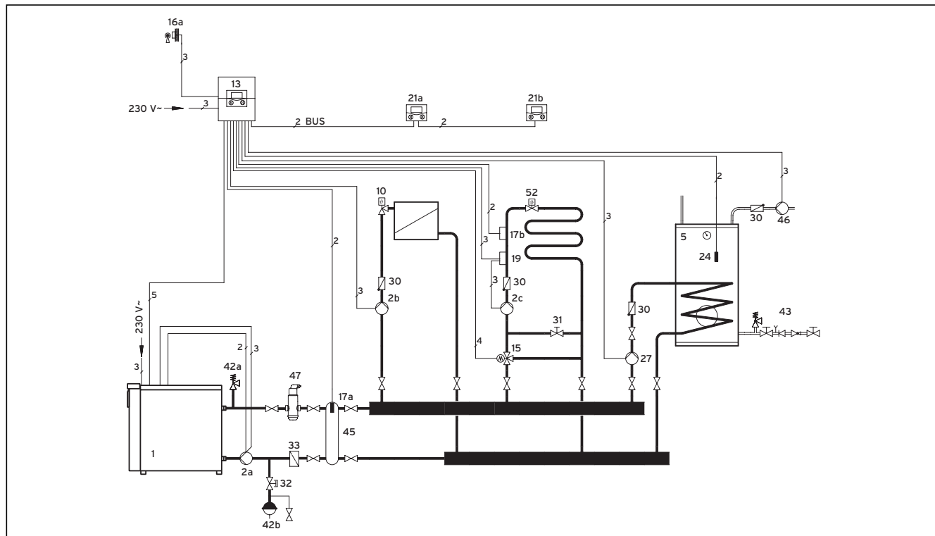
Рис. 4.1 Гидравлический план
