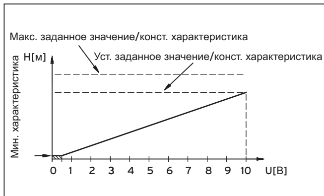
Рис. 7.2 Внешний аналоговый блок управления 0-10 В
